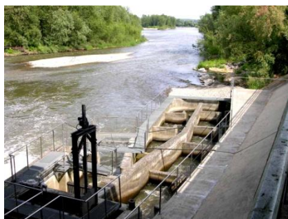
Рис. 6. Действующие рыбоходы в России (Нижнетуломский), Германии и Франции для пропуска лосося
